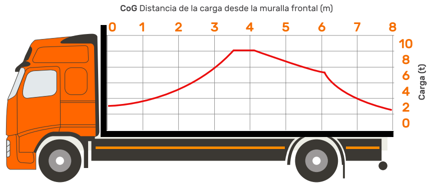
Diagrama de distribución de la carga en un camión de dos ejes
